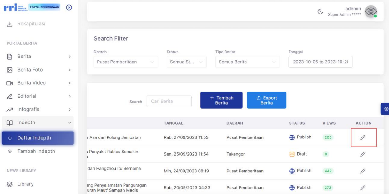
Gambar 12. Tombol Edit untuk Mengubah Data
